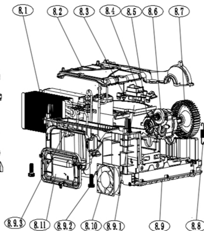
Base Subassembly
