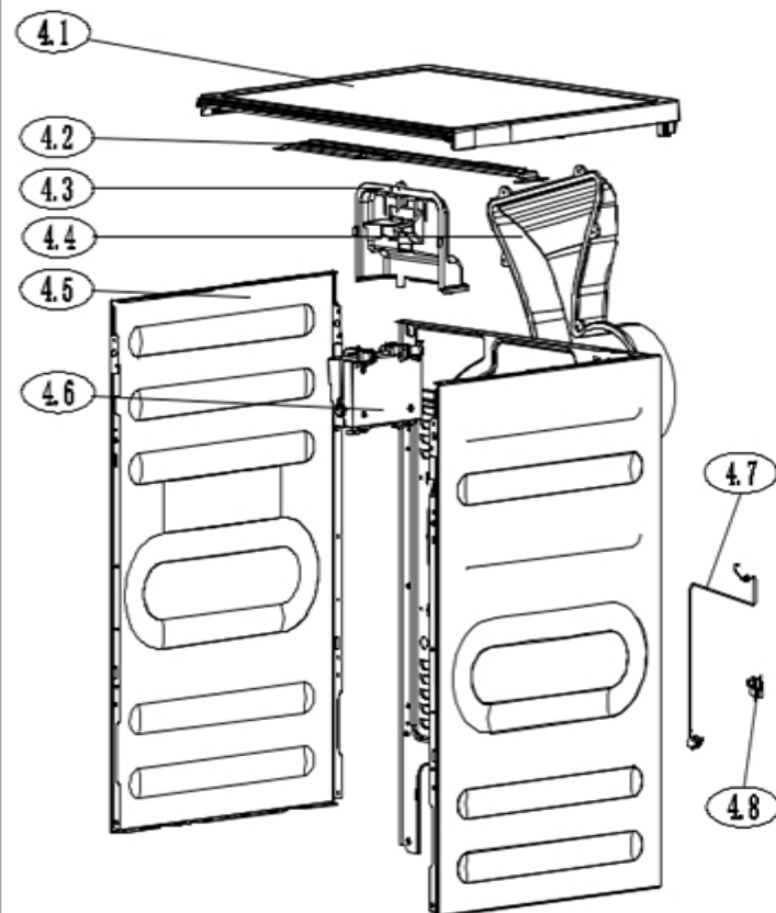
Cabinet Subassembly
