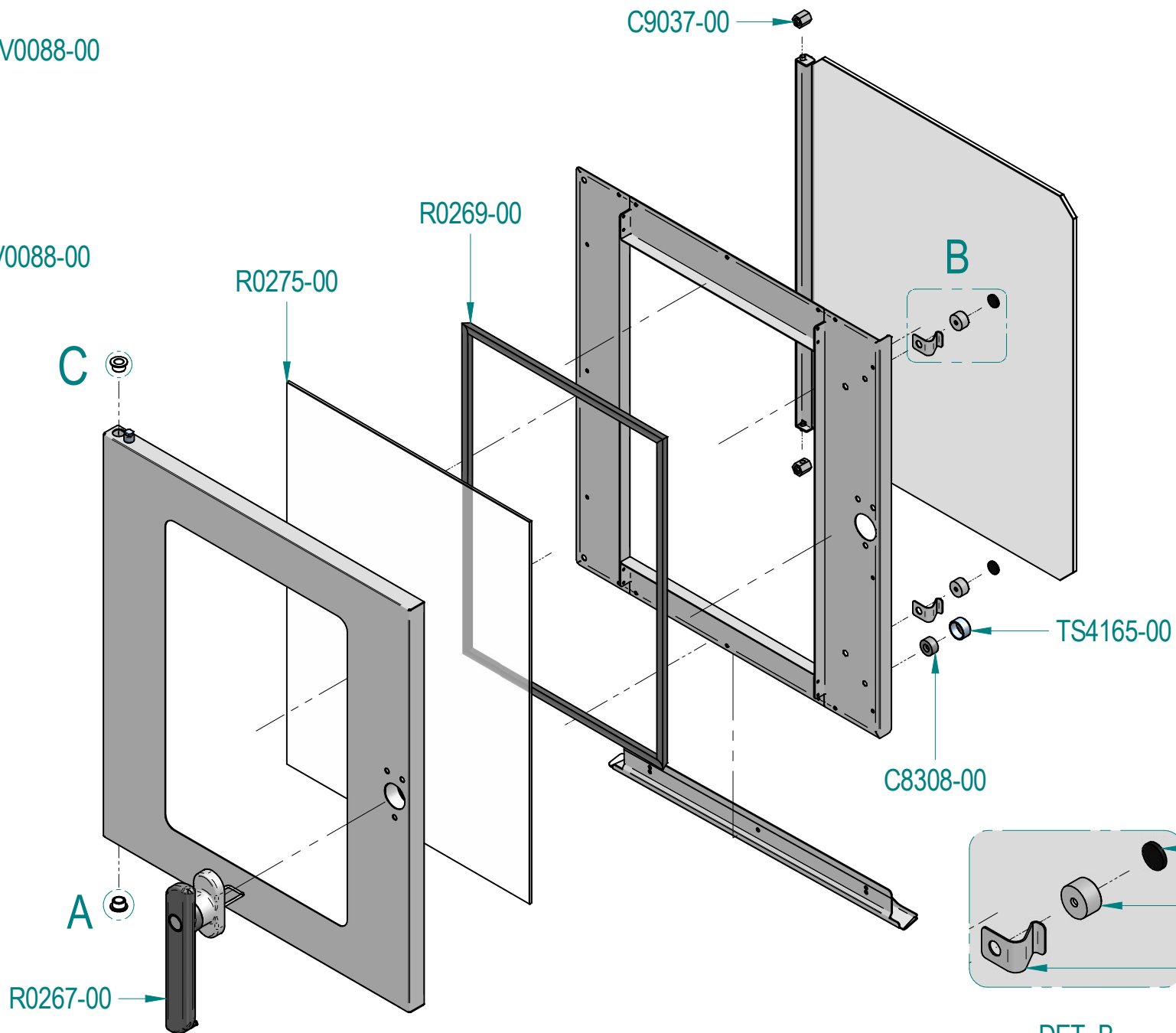
DET. B
