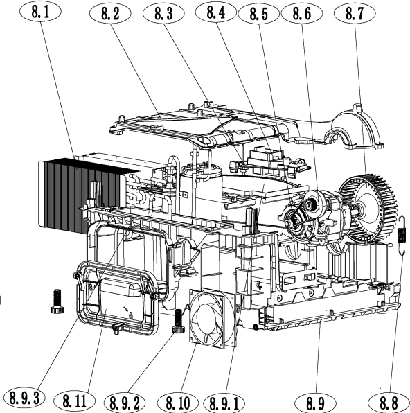
Base Subassembly
