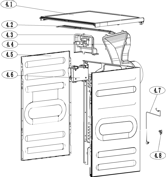
Cabinet Subassembly
