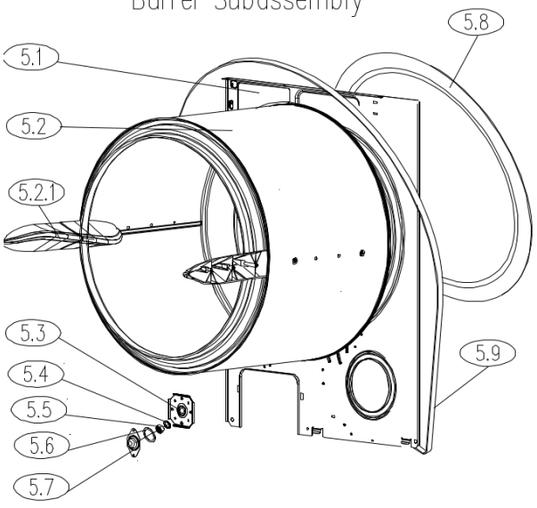
Barrel Subassembly
