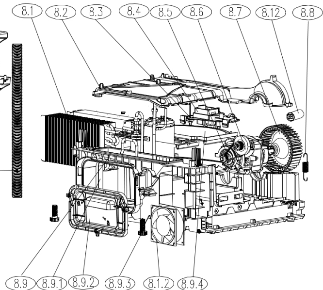
Base Subassembly
