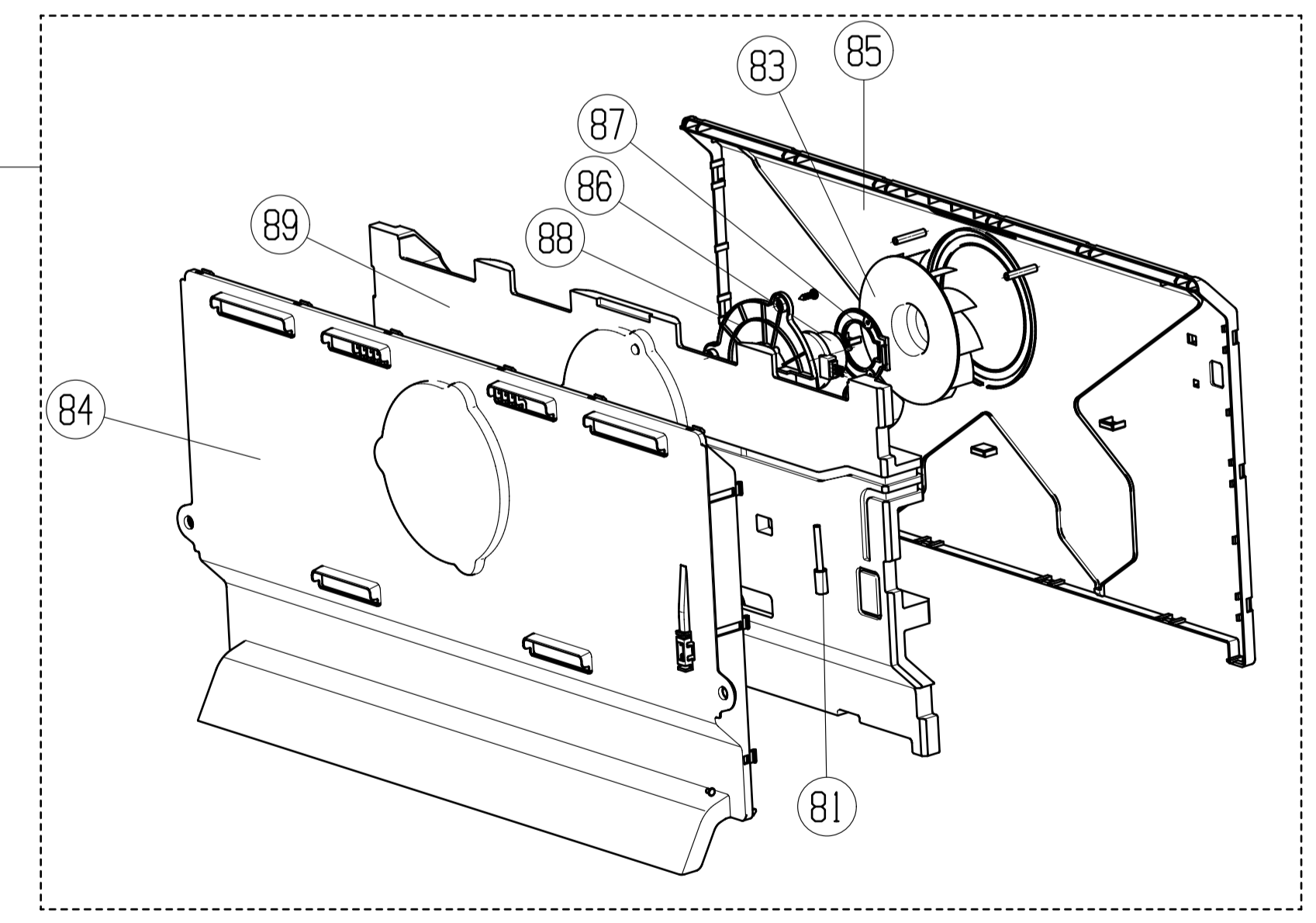
冷冻风道部件
