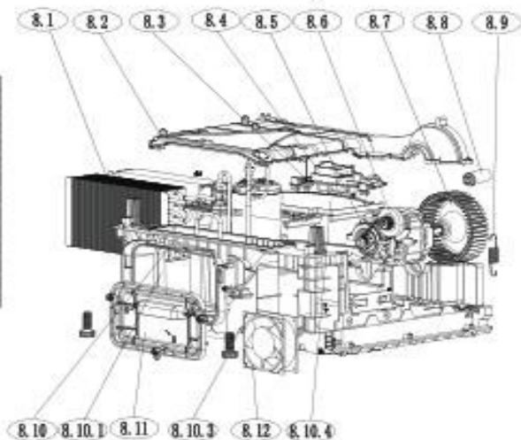
Base Subassembly
