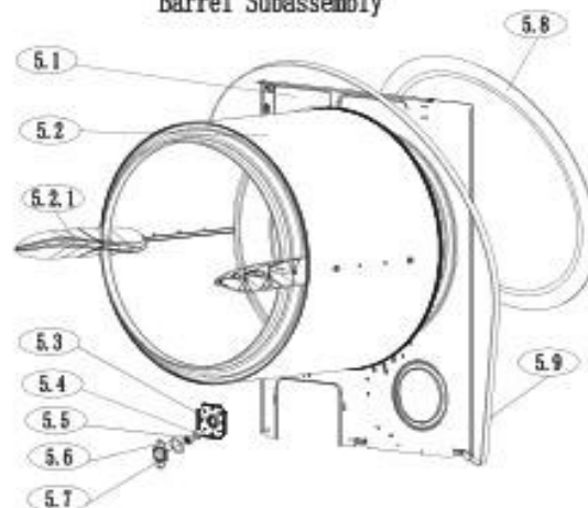
Barrel Subassembly
