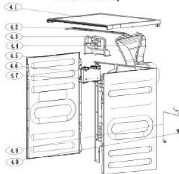
Base Subassembly
