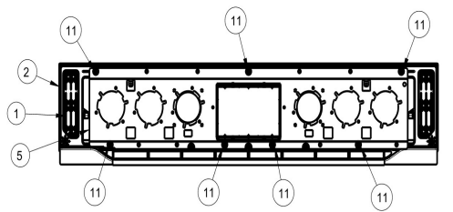
POSICIONES PARA EL ATORNILLADO DE LA MARCA 11 ESCALA 1/5
