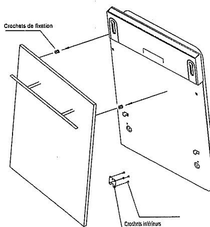
FIG 4a) Installation du panneau décoratif
