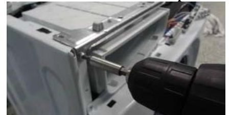
Enlever l'intercalaire de pompe
