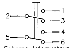
Schema Interrupteur
