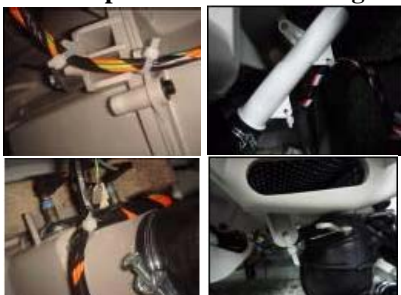
Enlever les clips de fixation amortisseur
