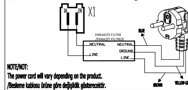
Power Cord&Parasite Filter Connection /Besleme Kablosu&Parazit Filtresi Bağlantıları
